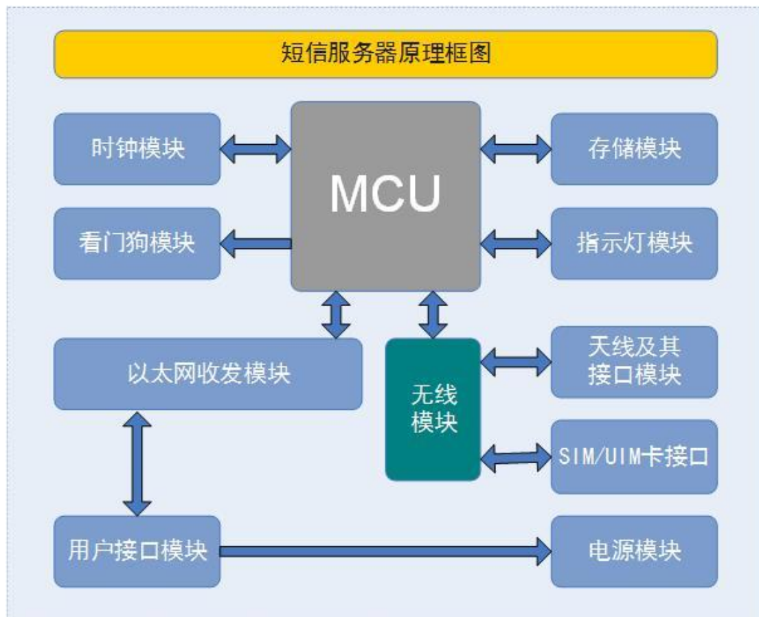
(图 2) 短信服务器原理框图
